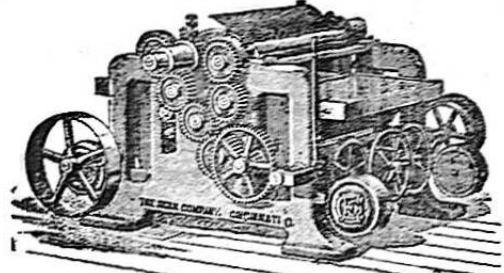
Cepillo y alisador reforzado n° 4.
