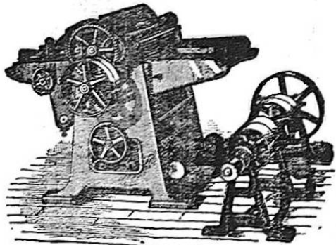
Cepillo y Machihembrador N° 2.
